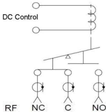
Volatge Control
